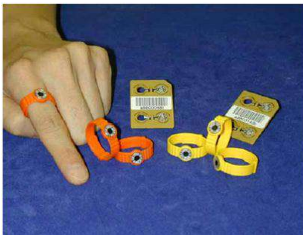
شکل ۸۷ - نمونه دزیمترهای ترمولومینسانس حلقه‌ای
