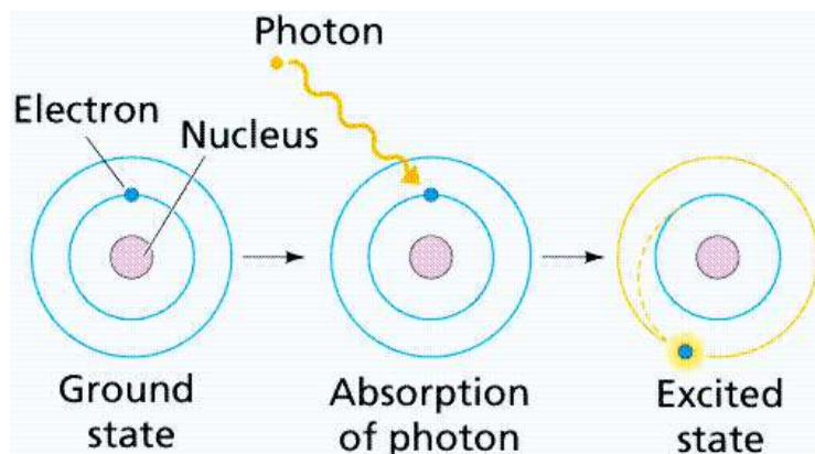
شکل ۵- نحوه تهییج اتم توسط پرتوهای فرابنفش
