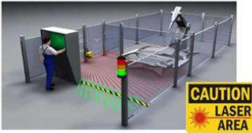
شکل ۷۱- جداسازی محل انجام عملیات صنعتی با استفاده از لیزر
