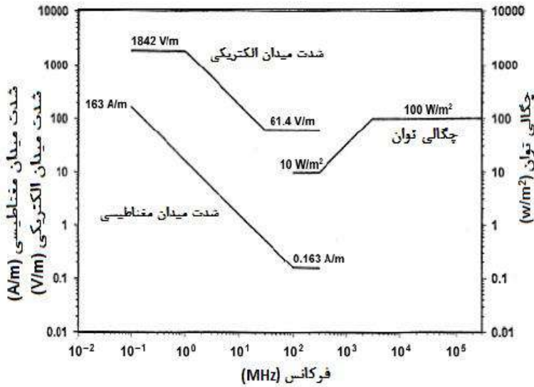
شکل ۵۲ - نمودار حد مجاز مواجهه شغلی امواج مایکروویو و رادیو فرکانسی (برای جذب ویژه تمام بدن کمتر از 0.4 \text{ W/kg} )
